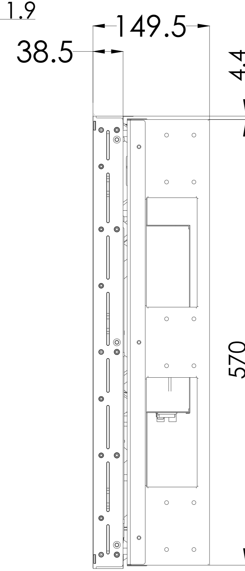
侧视图
