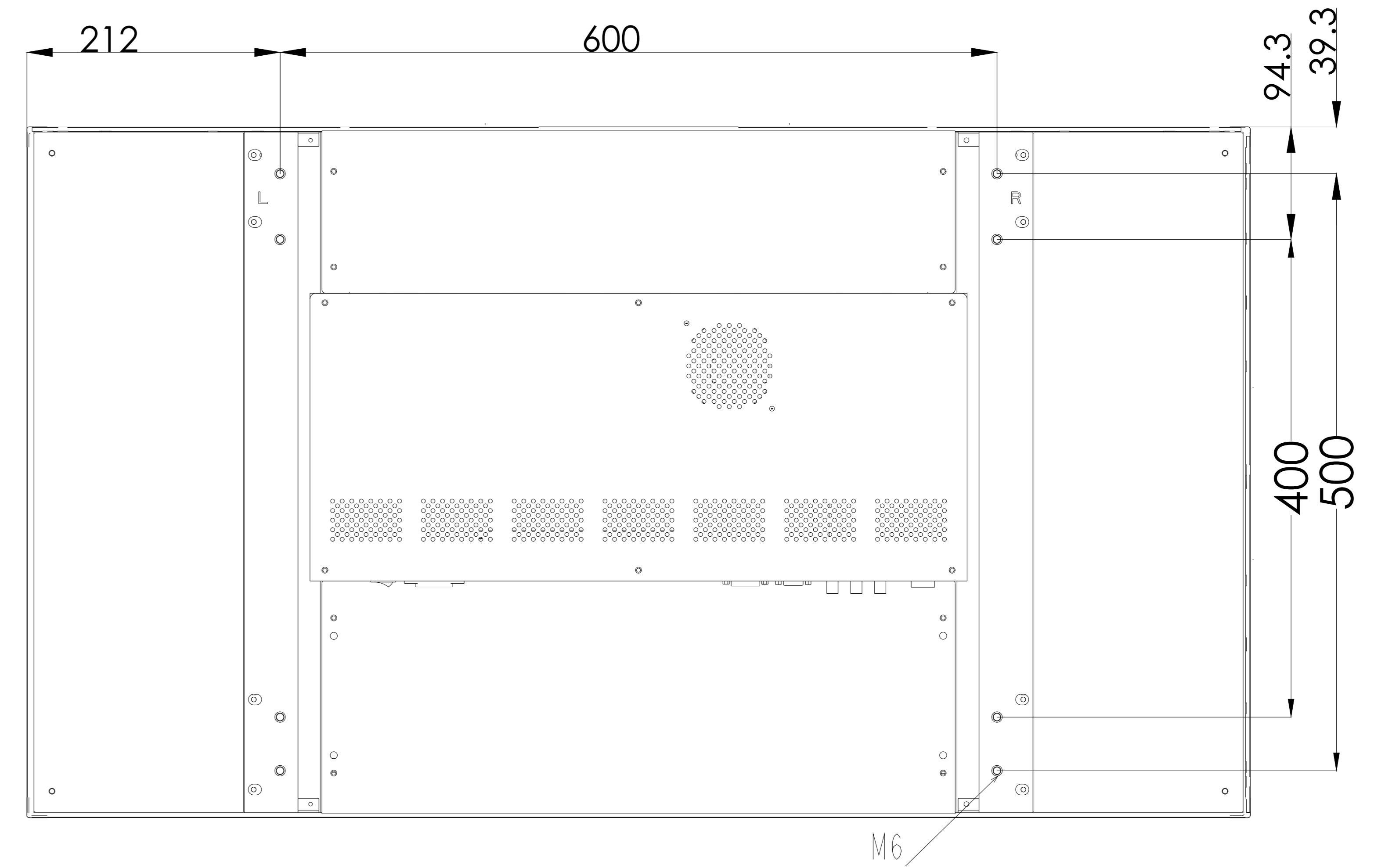
后视图
